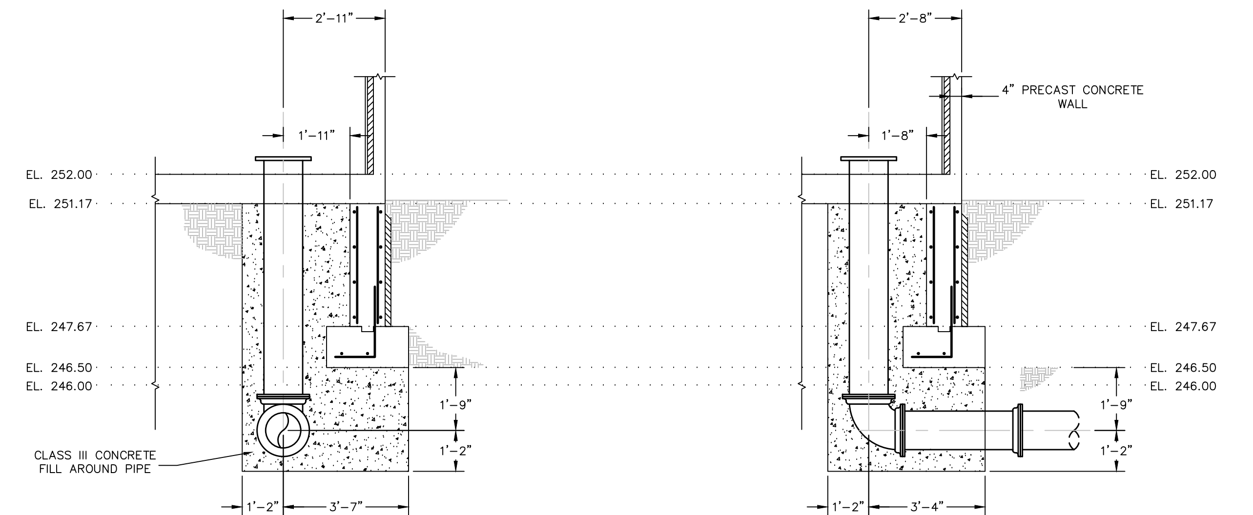
SECTION 3-3 SCALE: 3/8" = 1'-0"
