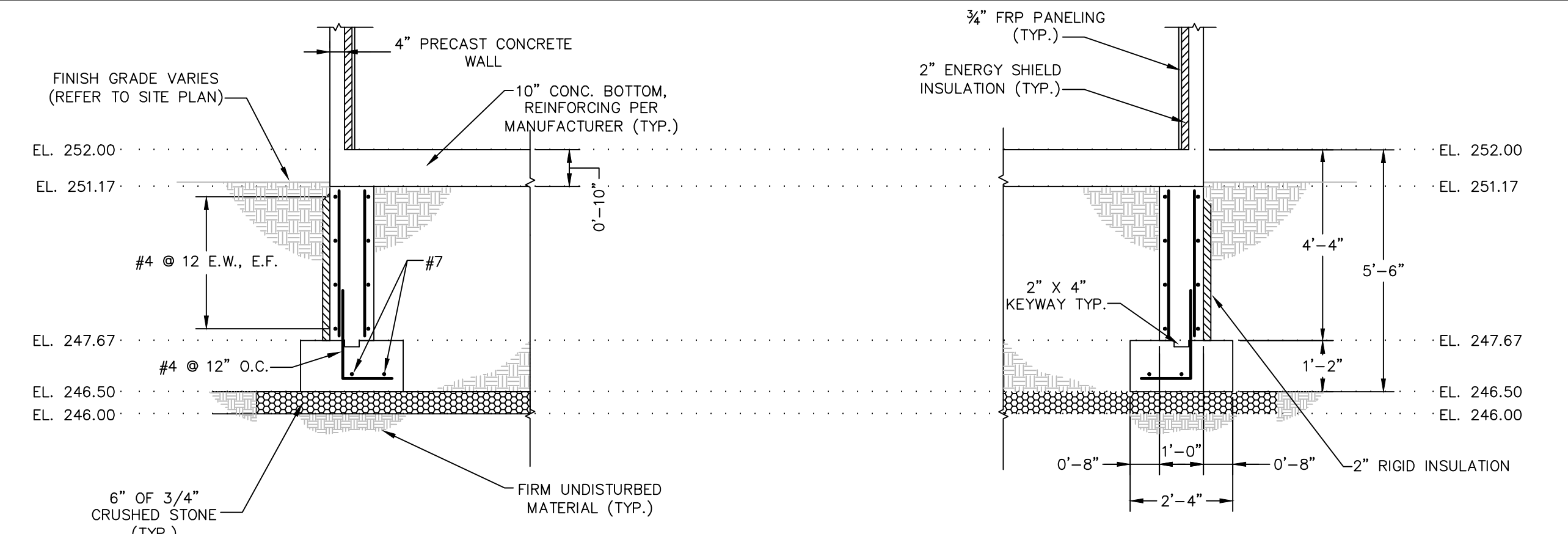
SECTION 1-1 SCALE: 3/8" = 1'-0"
